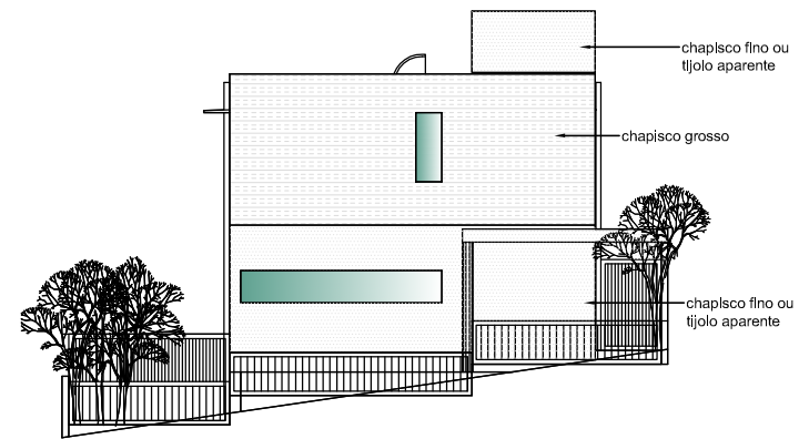
FACHADA LESTE esc1/100
