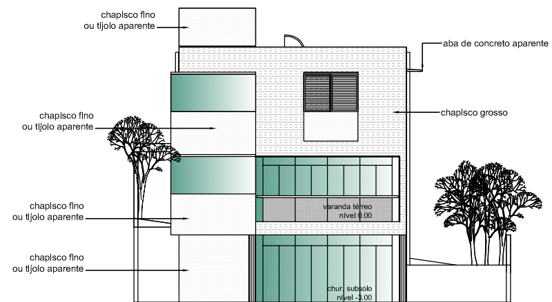
FACHADA OESTE esc1/100
